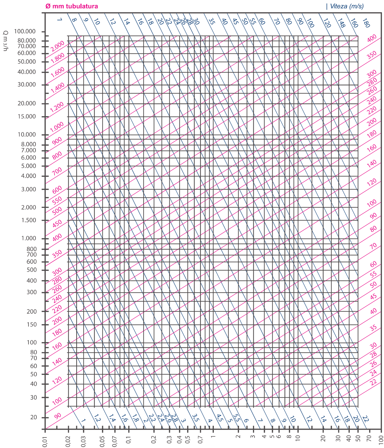
Pierdere de presiune \Delta p în mmCA pe 1 m ( \rho=1,2\text{Kg/m}^3 )
